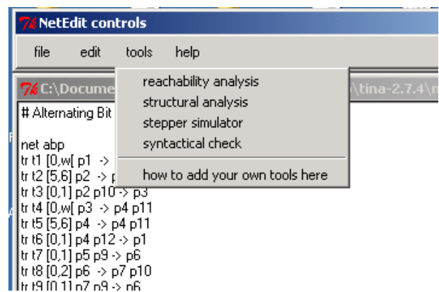
Fig. 4. Tina’s interface
